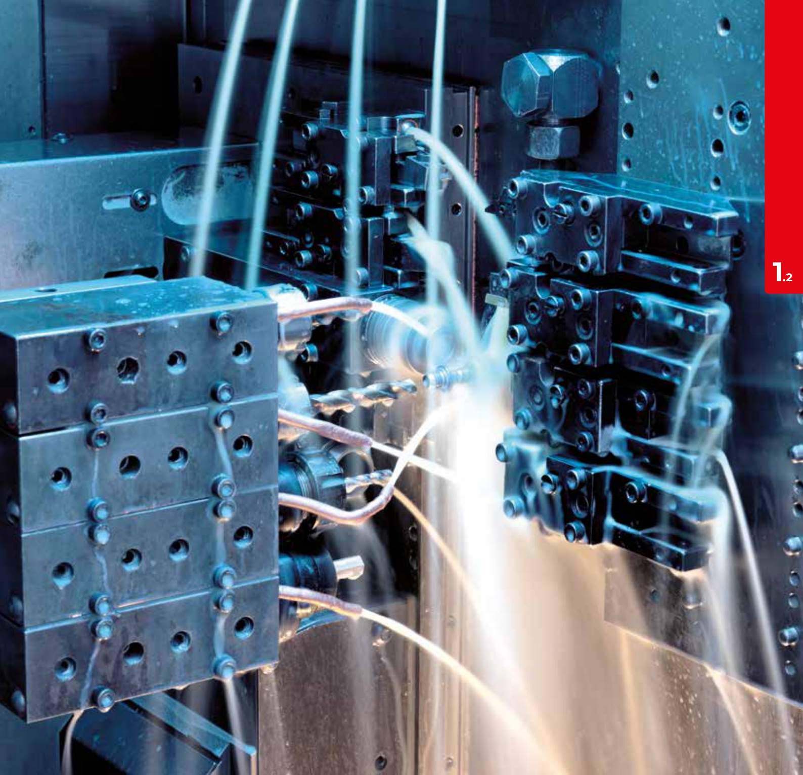
Particolare di una nostra macchina utensile: tornio CN a 10 assi ad alta precisione. One of our machine tools: CN lathe with 10 high-precision axes.
